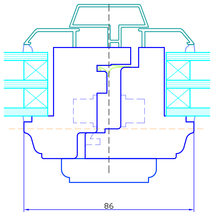
WK - Stulp mit Stulpgetriebe
