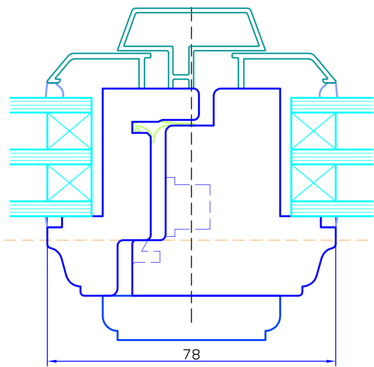
Standard-Stulp
